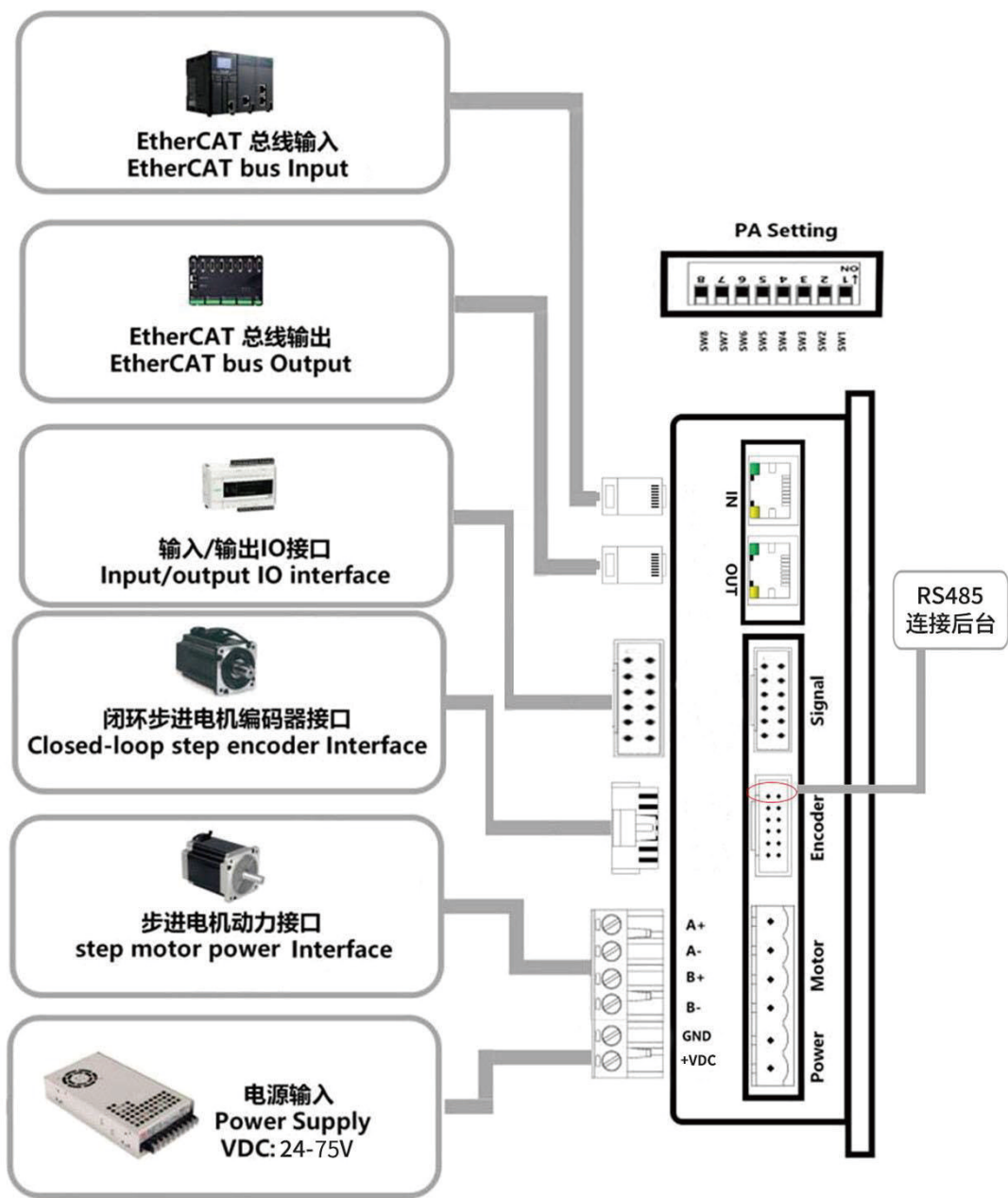
图 3-1 基本连接图
