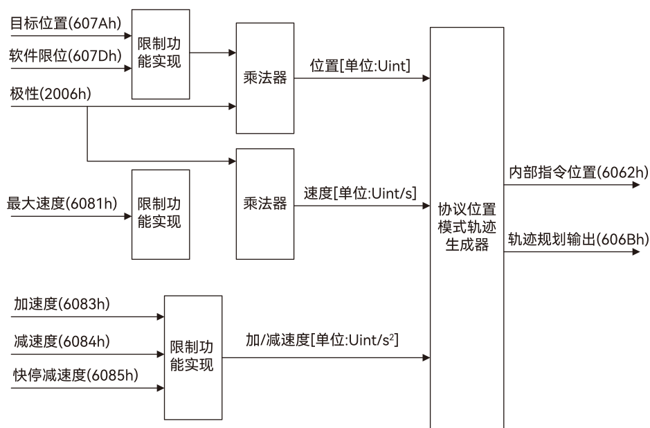
图 6-3 模式的轨迹生成
