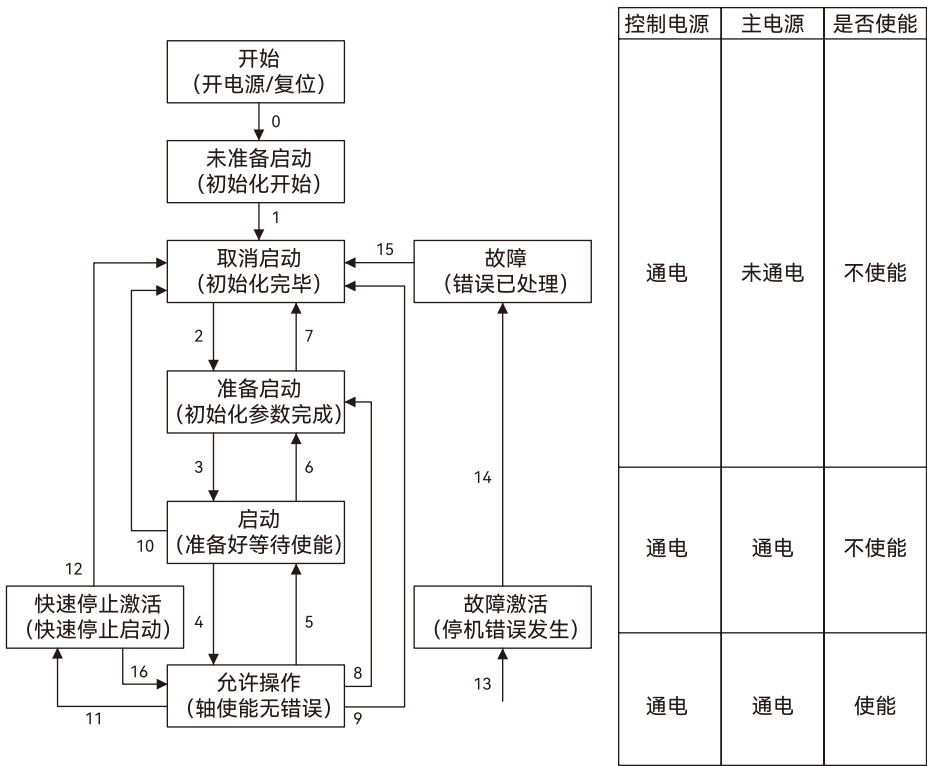
图 6-1 CIA402 状态机
