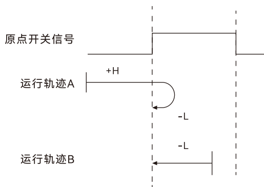
图 9-3 模式 19 原点回原运行轨迹示意图
