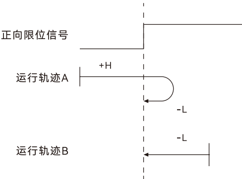
图 9-2 模式 18 原点回原运行轨迹示意图
