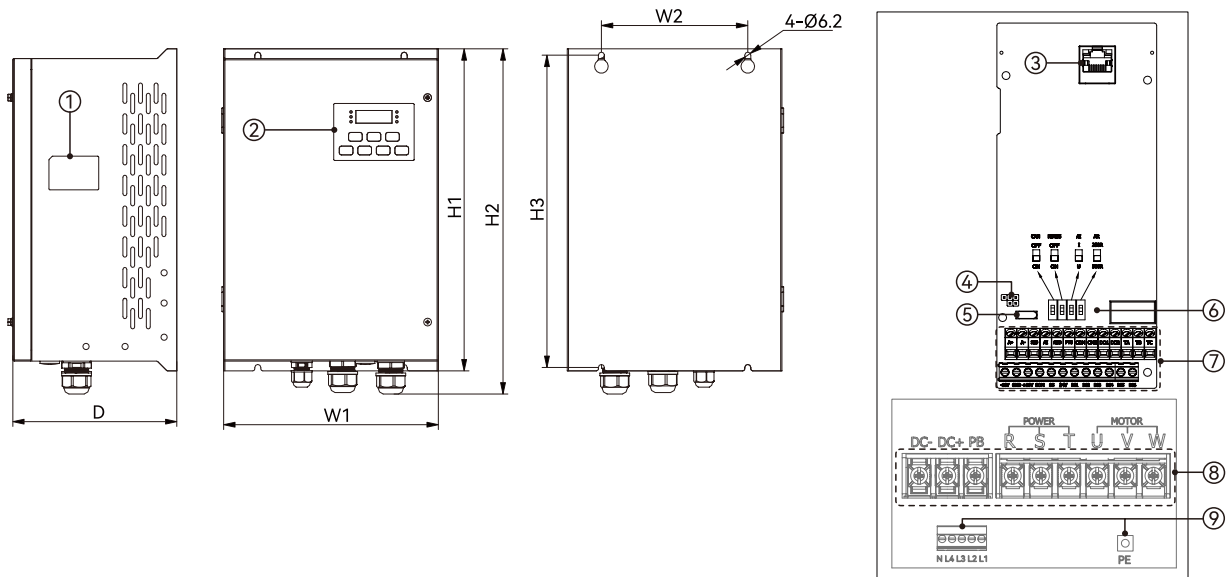
图 2-1 E615 系列尺寸接口示意图
