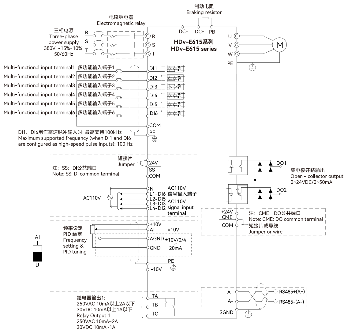
图 3-3 三相 380V 机种变频器标准接线图
