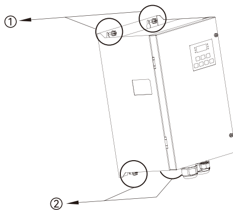
图 3-2 E615 整机拆装示意图
