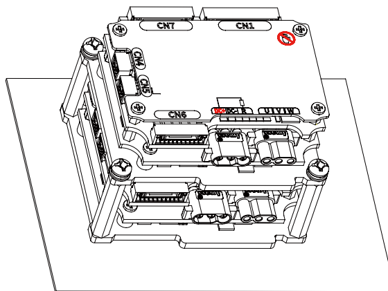
叠式安装
