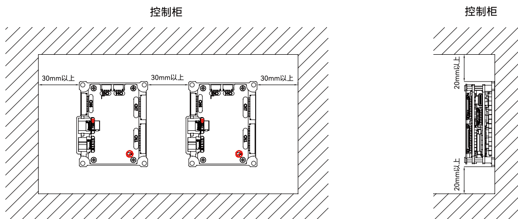
图 1. 驱动器的安装间隔图
