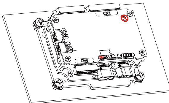
单机安装
