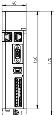
正视图
