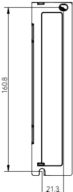
后视图
