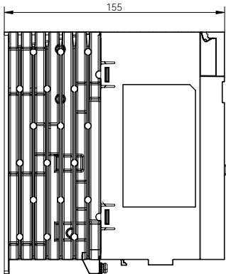
左视图
