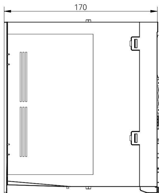
右视图
