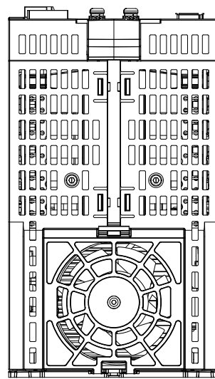
仰视图
