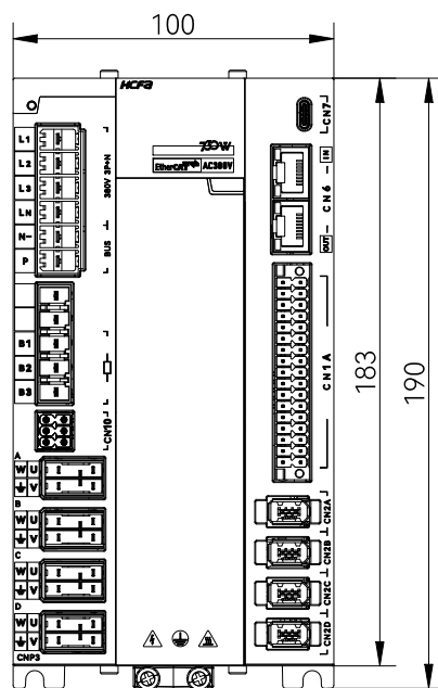
正视图
