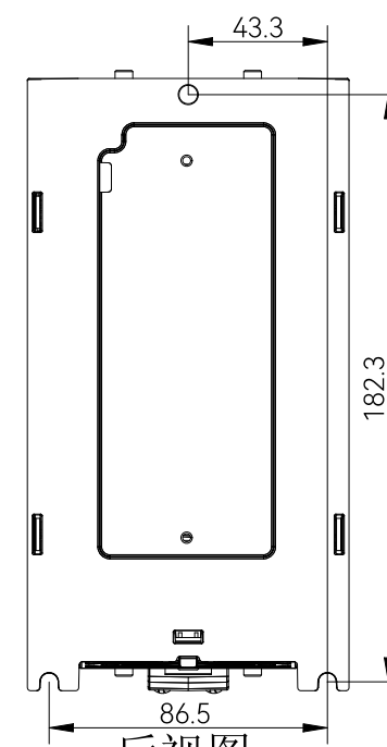
后视图
