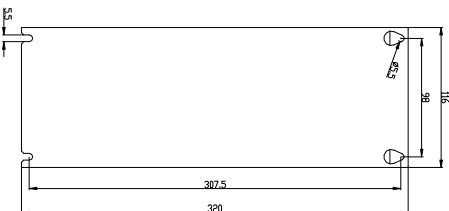
安装孔位图
