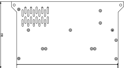
左视图
