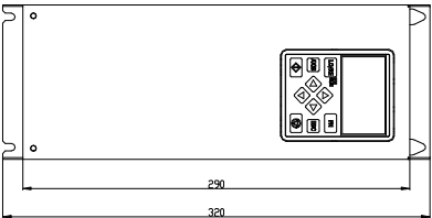
正视图
