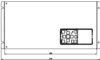
正视图
