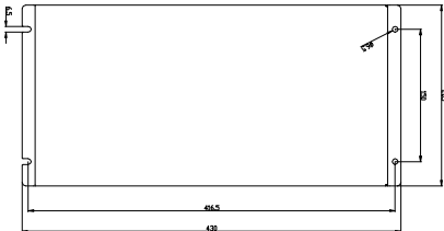
安装孔位图
