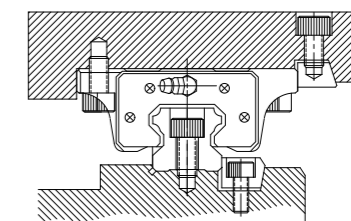
(d) 侧面使用楔形块固定
