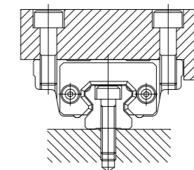
(d) 侧面使用使用定位销固定
