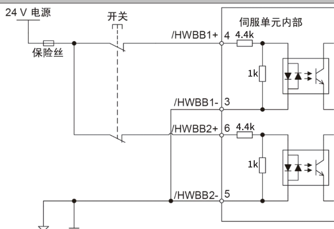
输入信号连接示例
