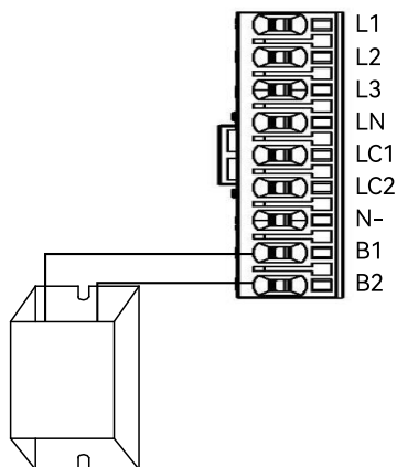
图 20. SIZE A 再生电阻连接
