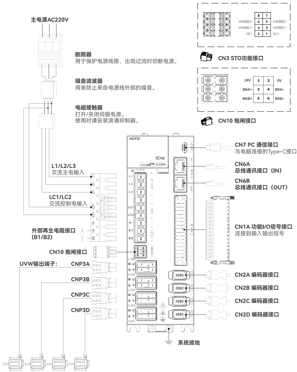
图 2. SIZE A AC220V(1P/3P) 伺服单元各部分介绍图
