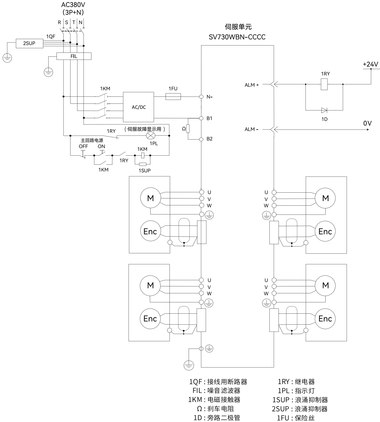
图 18. DC310V 输入型 SV730WBN-CCCC 接线
