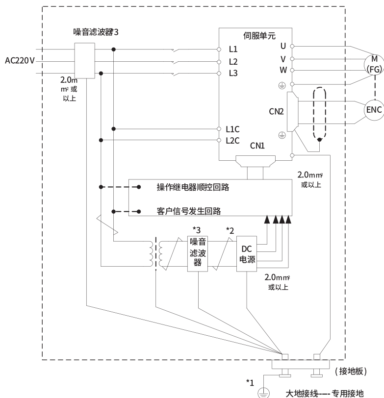
图 31. 噪音对策的接线示例图
