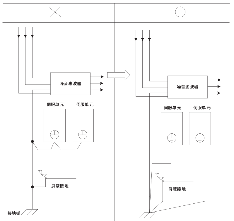
图 34. 噪音滤波器接地图
