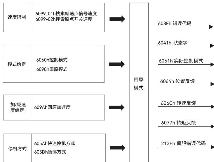
图 55. 原点模式输入输出
