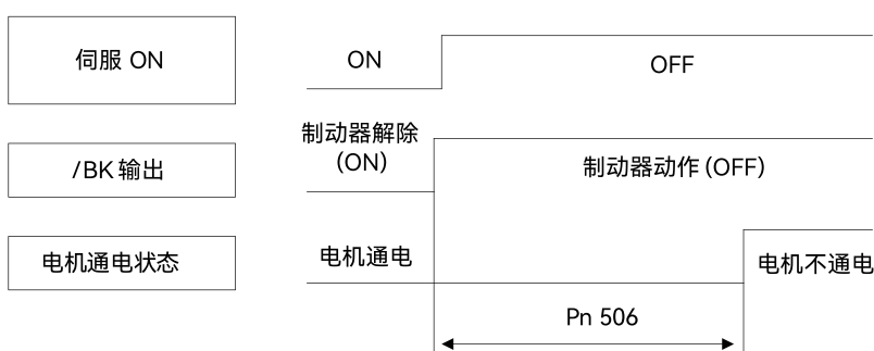
图 43. 制动器信号（/BK）的输出时序图（电机停止时）
