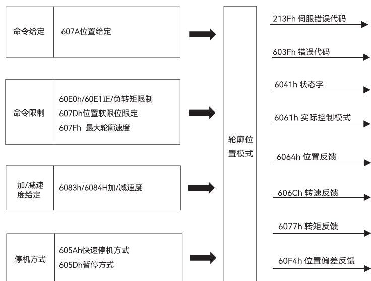
图 49. 轮廓位置模式输入输出
