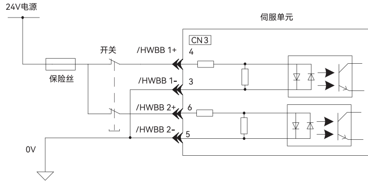
图 104. HWBB 输入信号连接示例图
