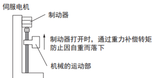
图 97. 功能运行图
