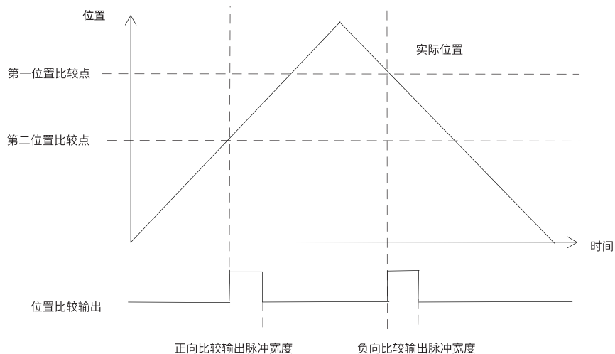
图 96. 功能运行图
