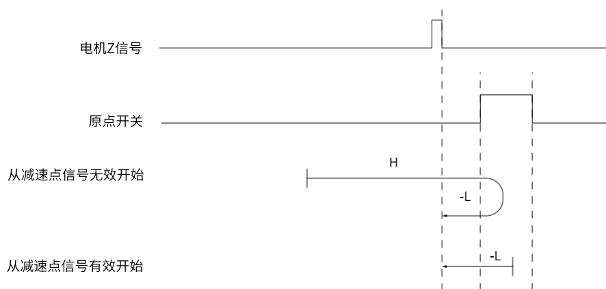
图 59. 原点模式 3 轨迹及信号状态
