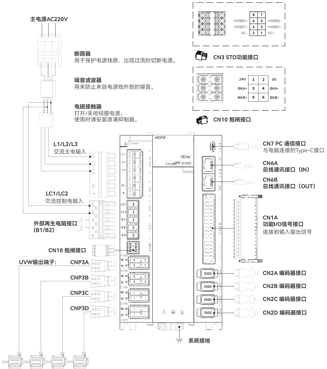
图 4. SIZE B AC220V(1P/3P) 伺服单元各部分介绍图
