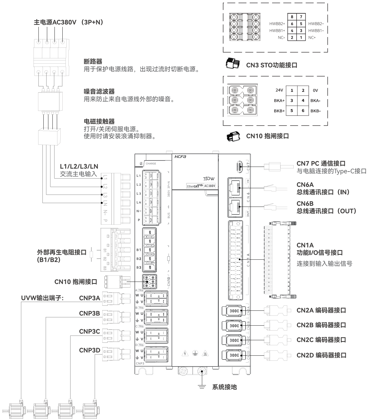
图 5. SIZE B AC380V(3P+N) 伺服单元各部分介绍图
