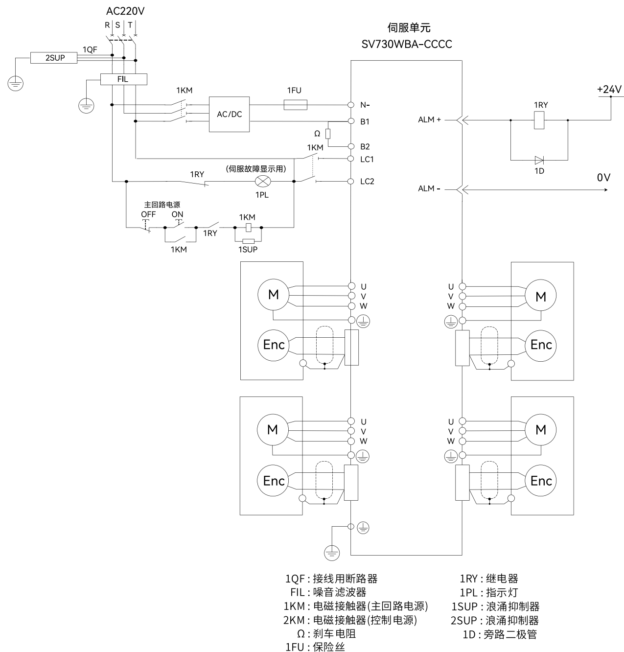
图 16. DC310V 输入型 SV730WBA-CCCC 接线
