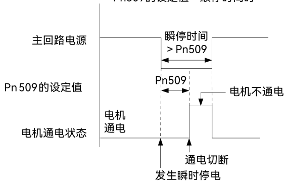
图 47. 主回路电源和电机通电状态图 (Pn509 的设定值 < 瞬停时间)
