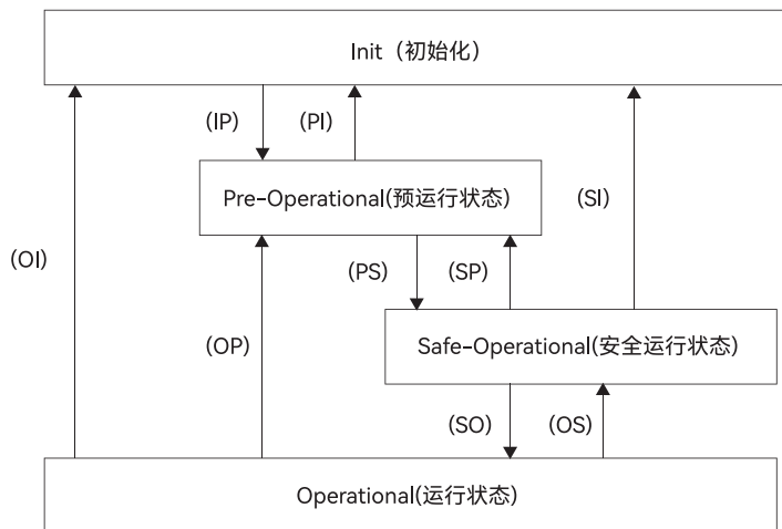
图 37. EtherCAT 状态机
