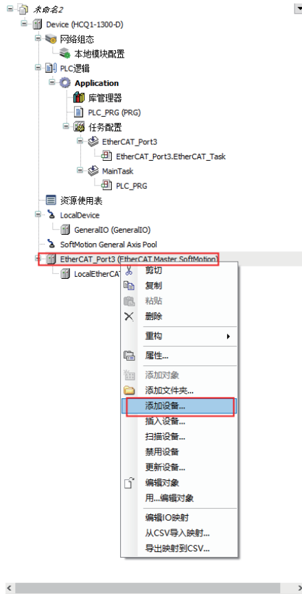
图 117. 添加设备
