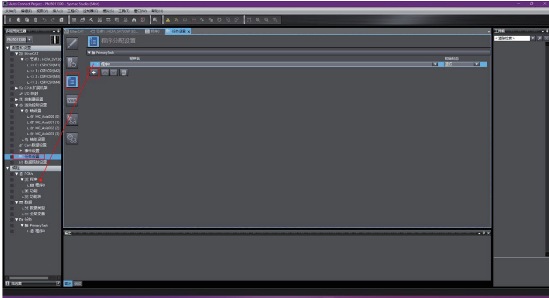
图 140. 添加程序名
