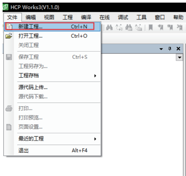
图 112. 新建工程
