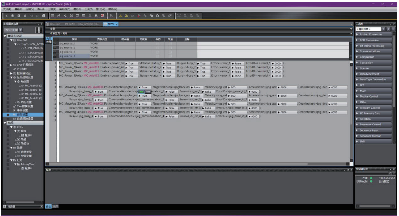
图 143. 运行
