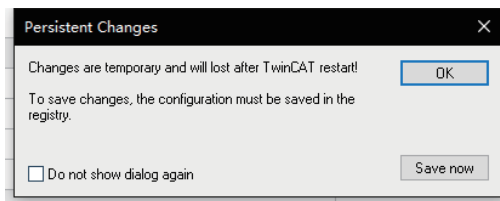
图 151. 参数下载
