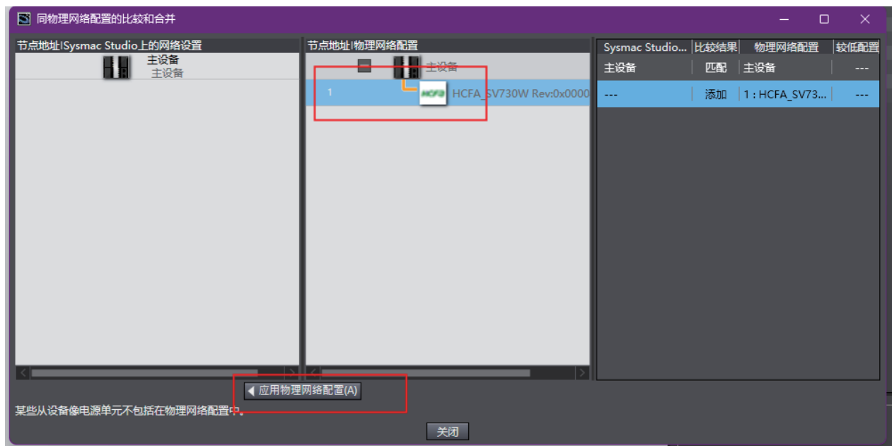
图 130. 添加 730W
