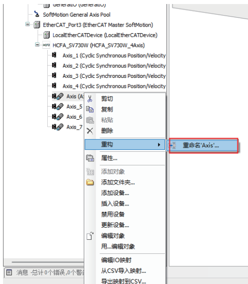
图 121. 重命名
