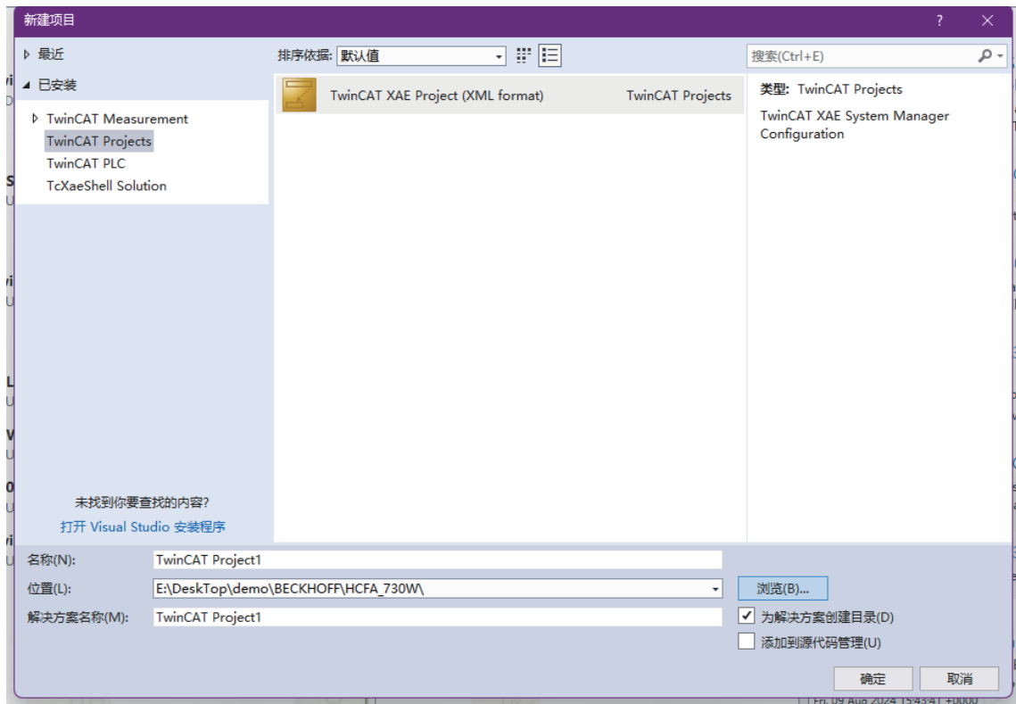
图 145. 新建方案
