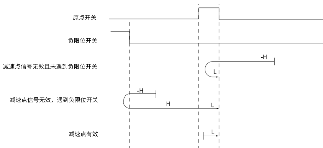
图 81. 原点模式 27 轨迹及信号状态
