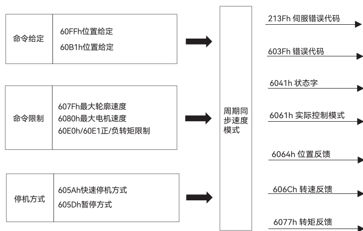
图 91. 周期同步速度模式输入输出
