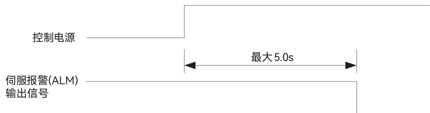
图 12. 伺服报警输出信号时序图
