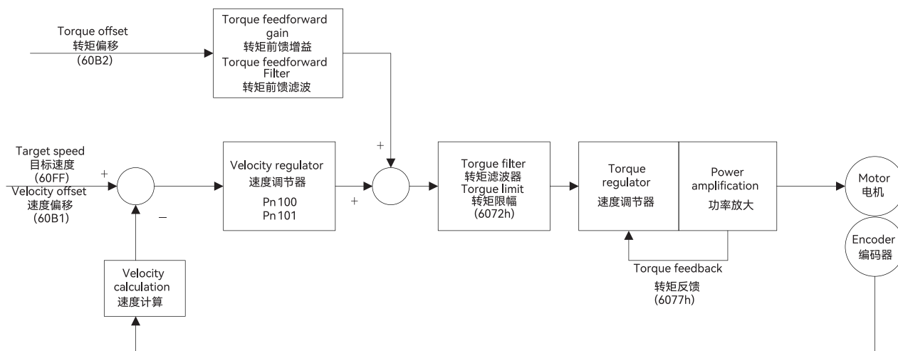
图 91. 周期同步速度模式输入输出
