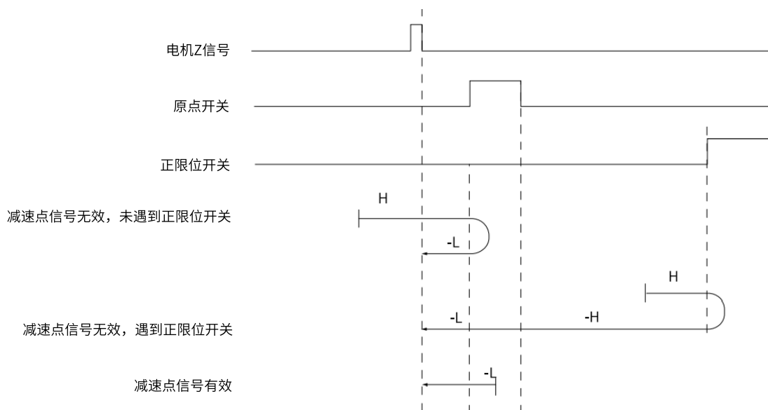
图 63. 原点模式 7 轨迹及信号状态
