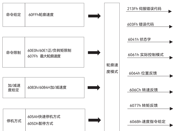
图 51. 轮廓速度模式输入输出
