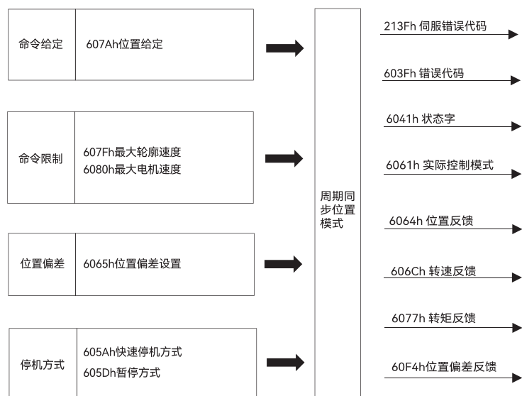
图 89. 周期同步位置模式输入输出
