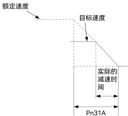
图 45. 减速停车的减速时间示意图
