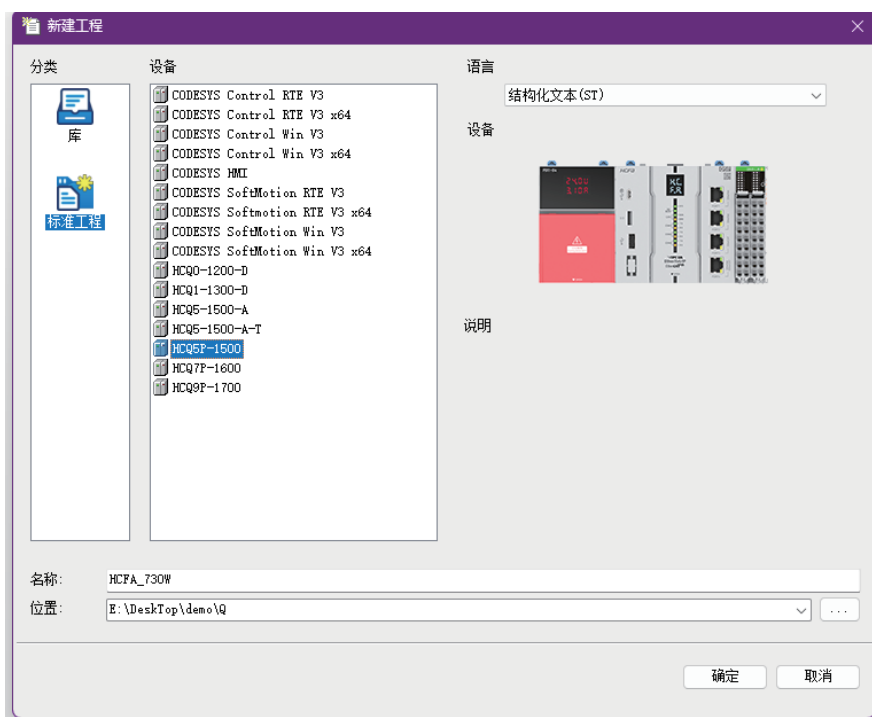
图 113. 工程详细
