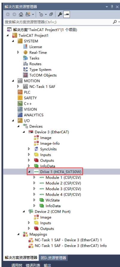
图 148. 扫描完成
