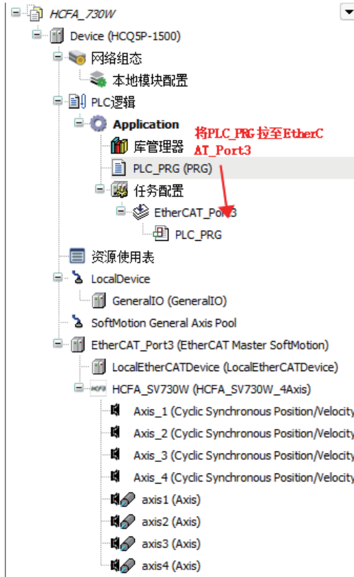
图 126. 移动 PLC_PRG(PRG)
