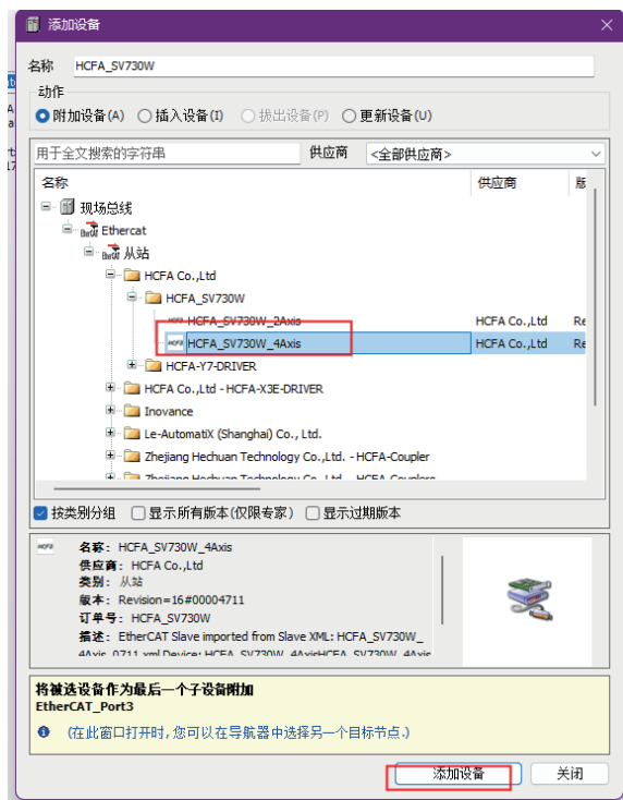
图 118. 选择【HCFA_SV730W_4Axis】
