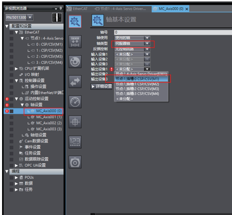
图 133. 添加伺服轴
