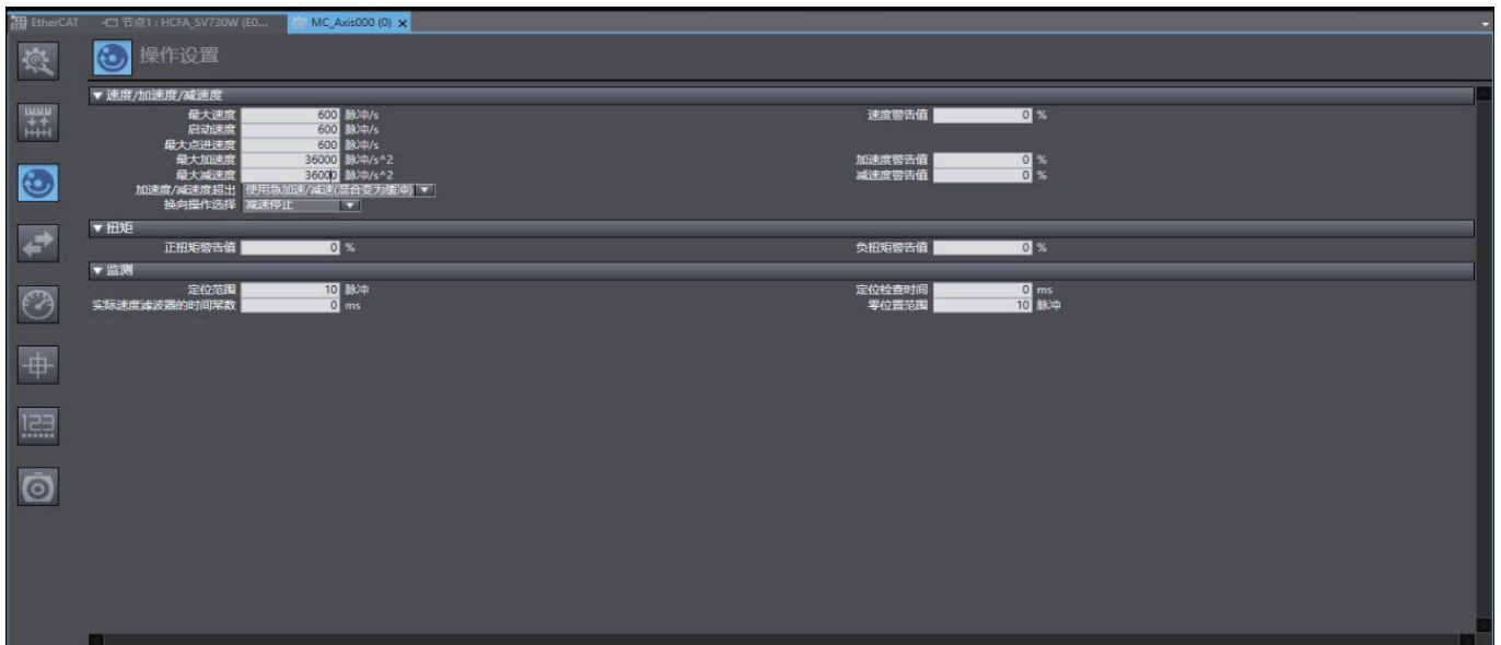
图 136. 设置速度
