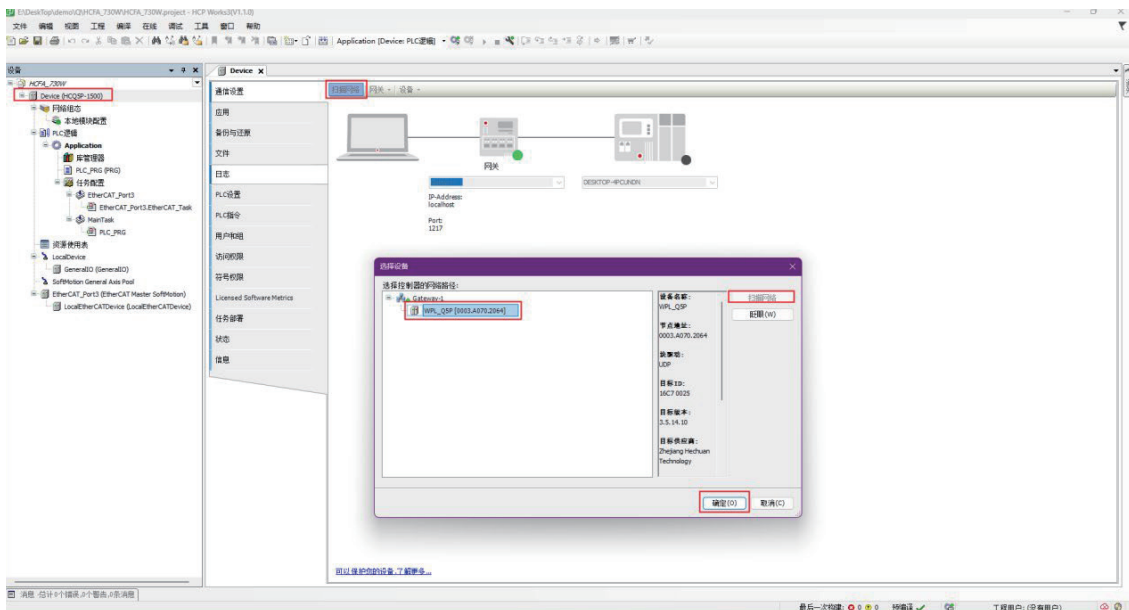
图 115. 网络连接
