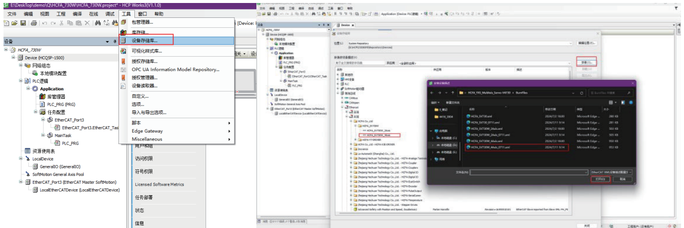
图 116. 添加 XML
