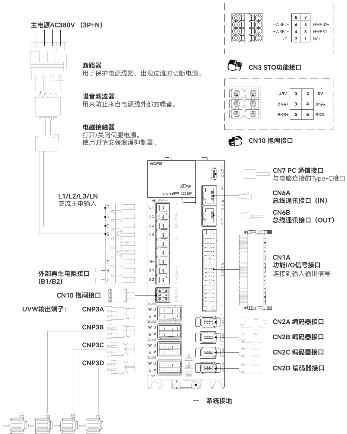
图 3. SIZE A AC380V(3P+N) 伺服单元各部分介绍图
