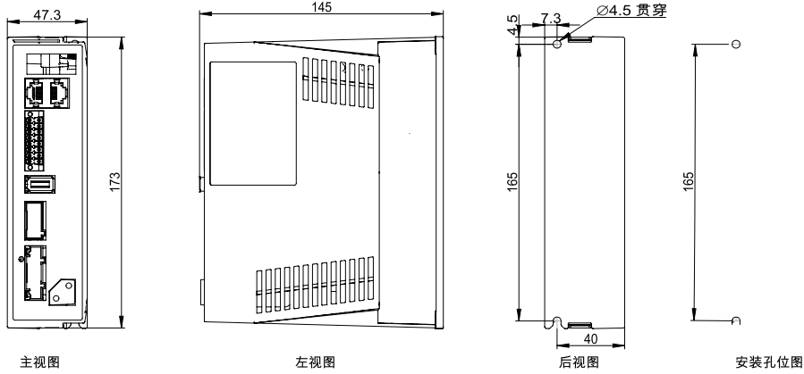
HY-A2004/HY-A2006驱动器外形尺寸
