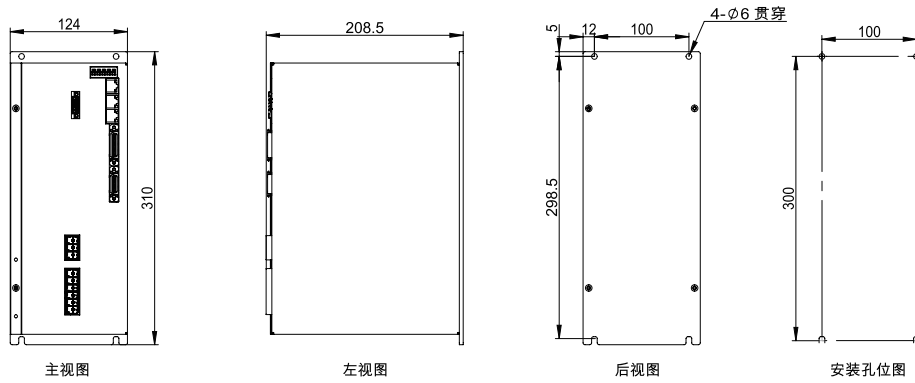
高压HY-A3030驱动器外形尺寸
