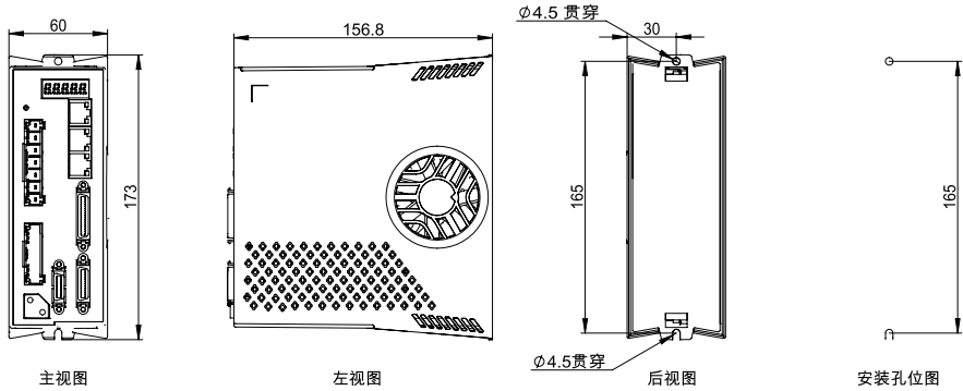
中压HY-A2008/HY-A2010/HY-A2013驱动器外形尺寸
