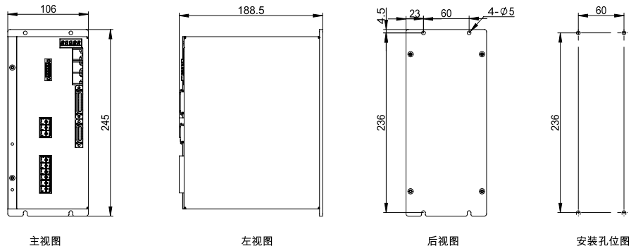
高压HY-A3024驱动器外形尺寸
