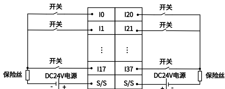
图 11 数字量输入模块外部接线图
