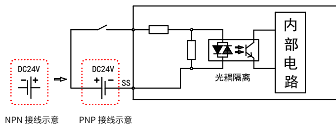
图 10 数字量输入模块内部电路图
