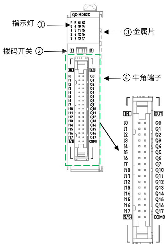
图 6 HCQX-MD32C-D2-□□□示意图
