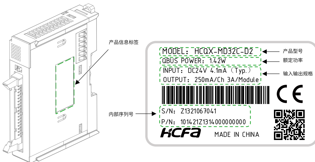
图1 模块型号与标签说明
