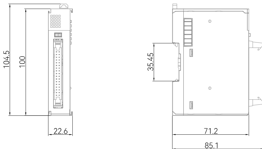
图9 HCQX-ID/OD/MD32C-D2-□□□□ 扩展模块安装尺寸
