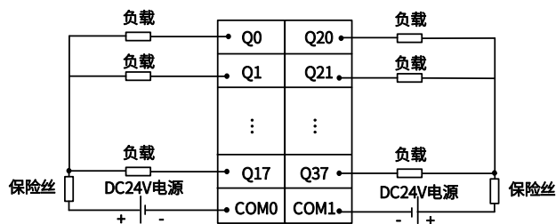
图 13 数字量输出模块（标准版本）外部接线图
