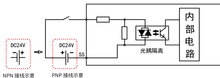
图 14 数字量混合模块（标准版本）输入内部电路图
