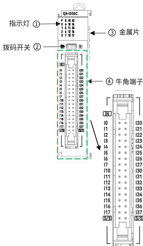
图2 HCQX-ID32C-D2 示意图
