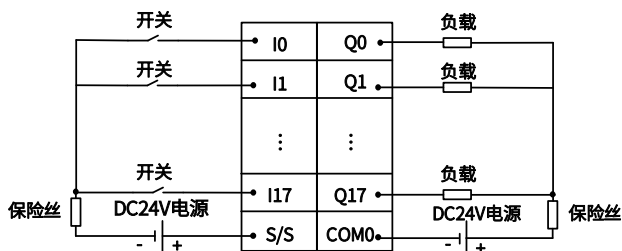
图 16 数字量混合模块（标准版本）外部接线图
