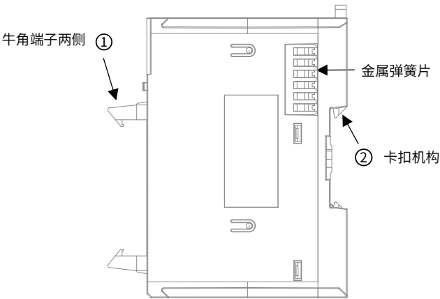
图 8 数字量模块侧视图
