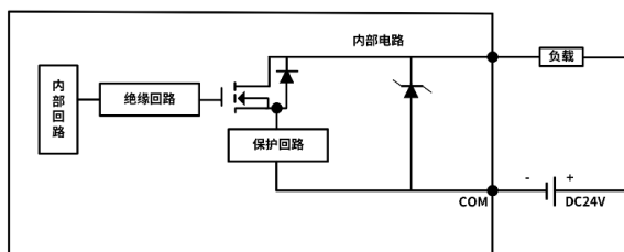
图 15 数字量混合模块（标准版本）输出内部电路图
