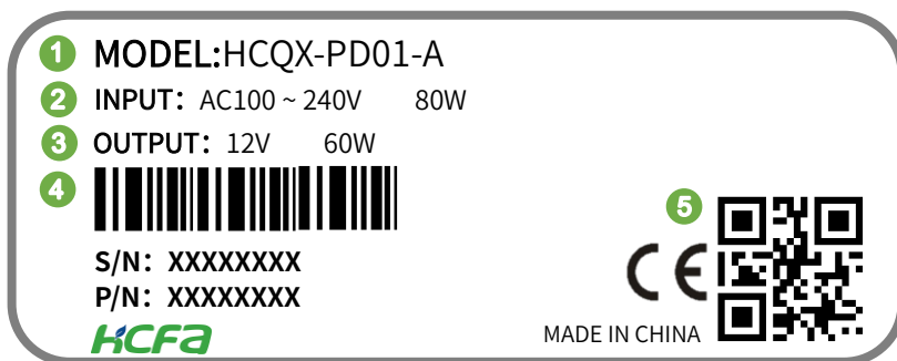
图 2 HCQX-PD01-A 型号与标签说明
