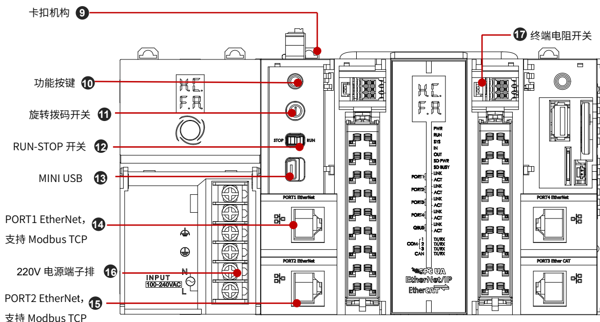
图 4 HCQ5-1500-A 正视图左侧说明图
