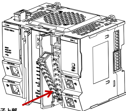
向内推动 IO 端子上部
