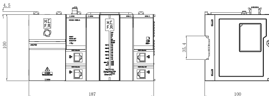
图9 HCQ5-1500-A CPU 模块安装尺寸 (单位: mm)
