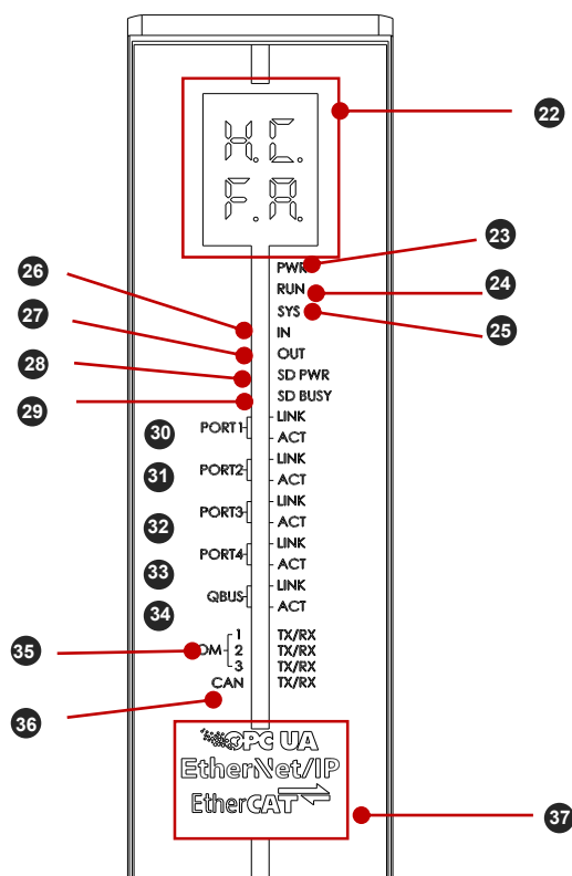
图 7 HCQ5-1500-A 指示灯说明图
