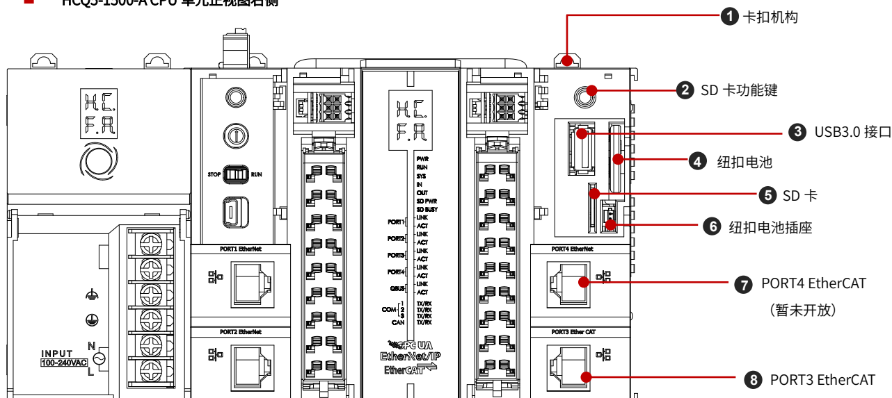
图3 HCQ5-1500-A 正视图右侧说明图
