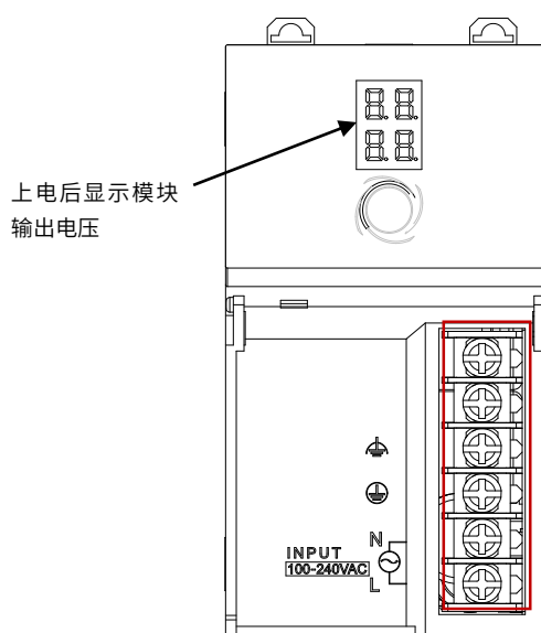
图 6 HCQ5-1500-A 电源模块说明图
