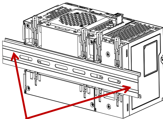
安装 35MM 国际导轨燕尾槽固定件
