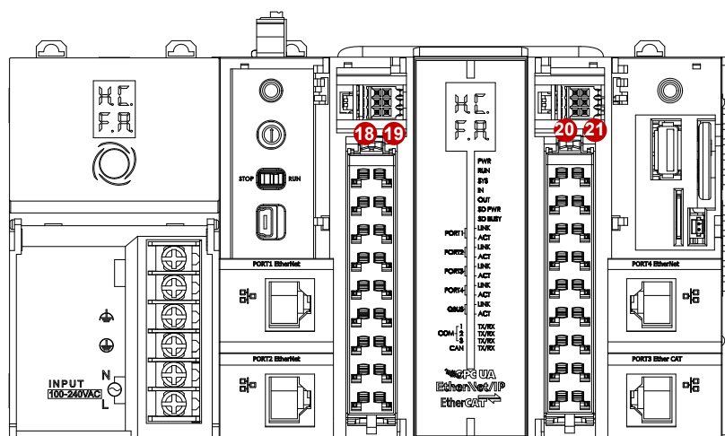
图 5 HCQ5-1500-A IO 接口及通讯接口说明图
