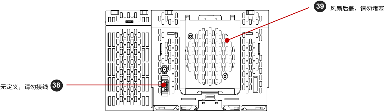
图 8 HCQ5-1500-A 俯视图说明图
