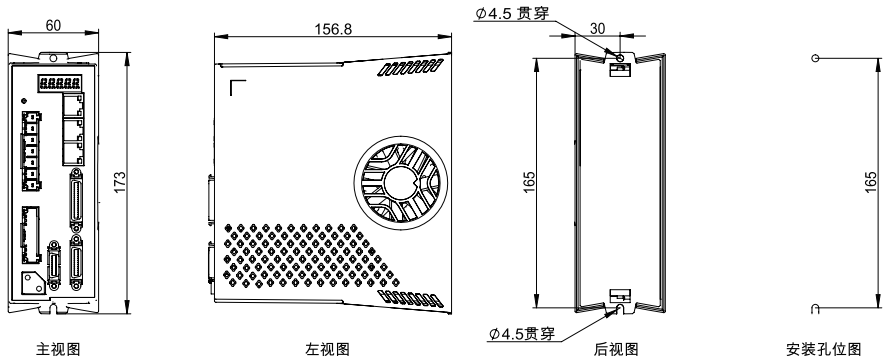
中压HY-A2008/HY-A2010/HY-A2013驱动器外形尺寸
