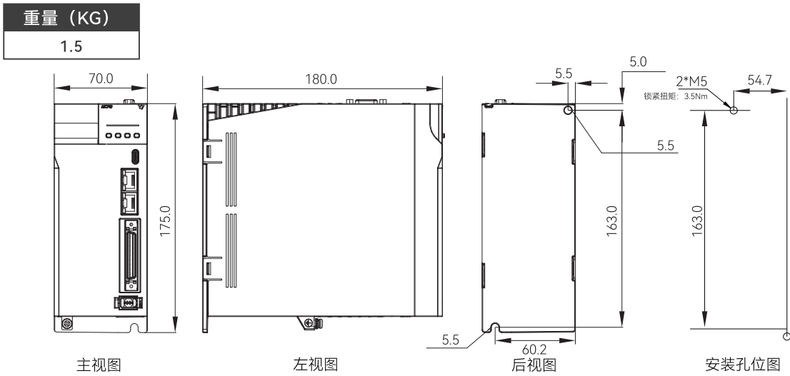
380V 5KW驱动器外形尺寸
